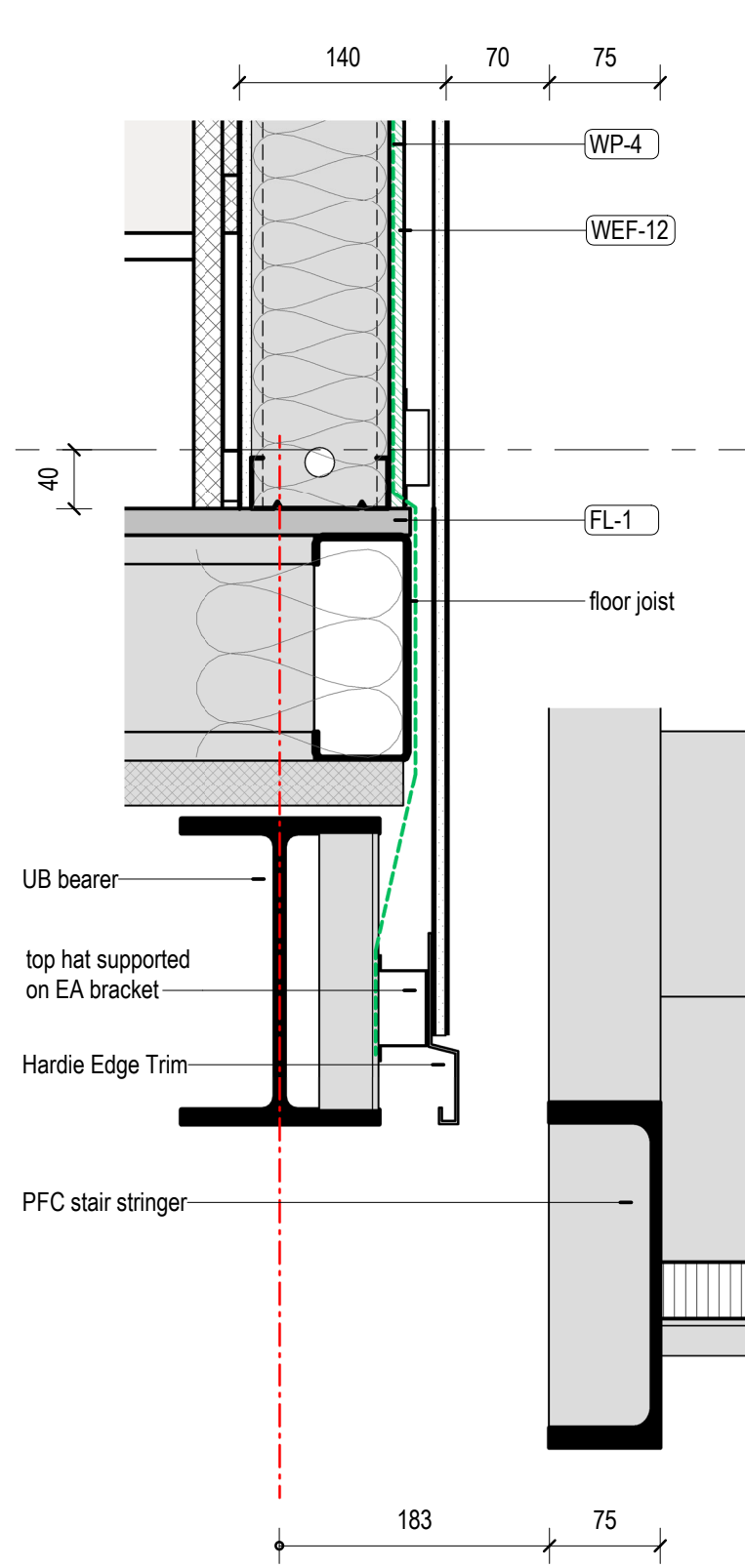
4 Stair 1 South Edge 1:5
