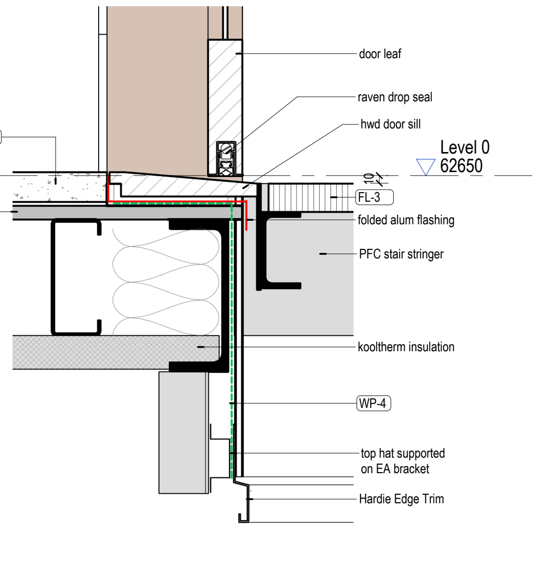
6 Stair 1 - Door Threshold 1:5
